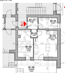
Bytová jednotka B1_1 PŮDORYS 1 NP
