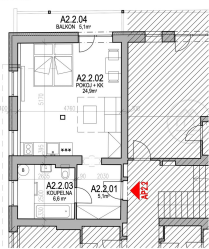
Apartmán AP2.2 PŮDORYS 2 NP
