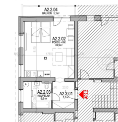
Apartmán AP2.2 PŮDORYS 2NP
